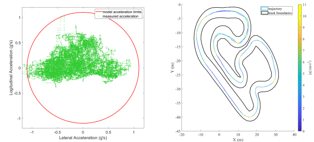
(a) G-G Circle
