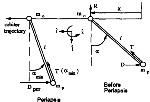
Fig. 9. Sliding pendulum.
